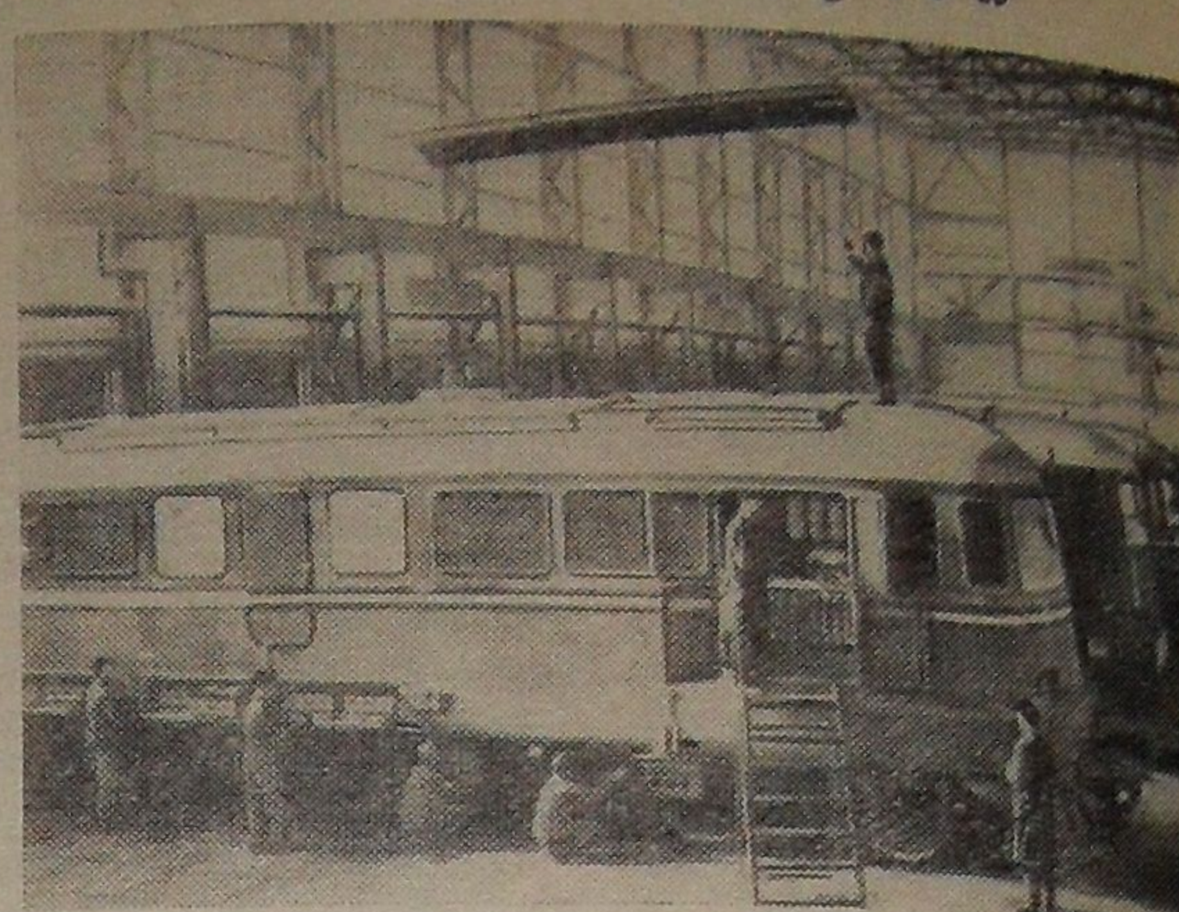
РУМЫНСКАЯ НАРОДНАЯ РЕСПУБЛИКА. Завод «Электротепло» в Крайове выпускает тепловозы мощностью 2.100 лошадиных сил. Из цехов предприятия вышли первые десяти тепловозов такого типа.
