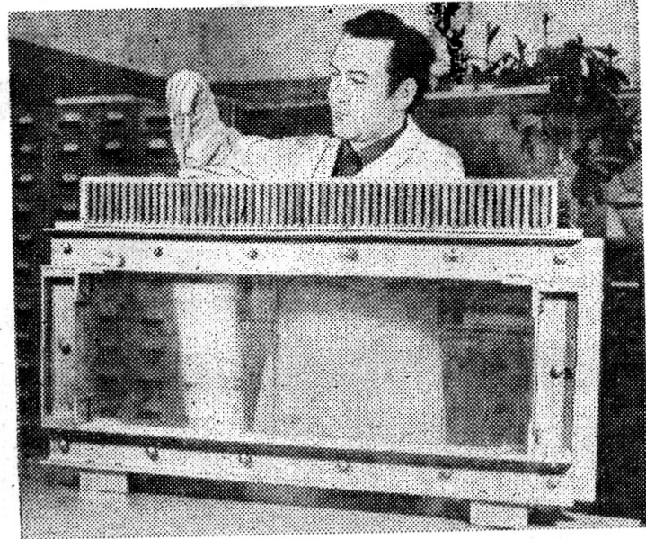
В секторе бесфильмовых камер Лаборатории высоких энергий разработаны пропорциональные камеры размером 900 мм x 300 мм (руководитель работ — старший инженер В. Д. Пешехонов).
