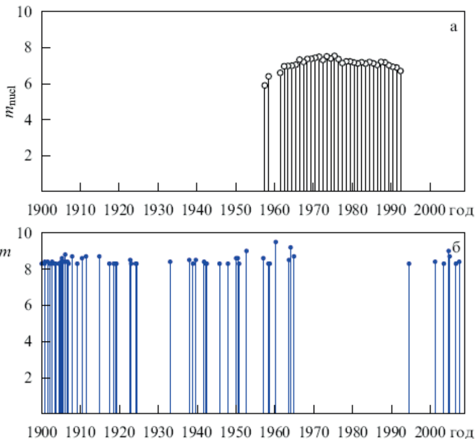
а) Ежегодная совокупная энергия подземных ядерных взрывов СССР и США, выраженная по шкале Гутенберга–Рихтера, в период 1957–1992 гг. б) Сильнейшие землетрясения с магнитудой m > 8,3 с 1900 по 2008 год.
