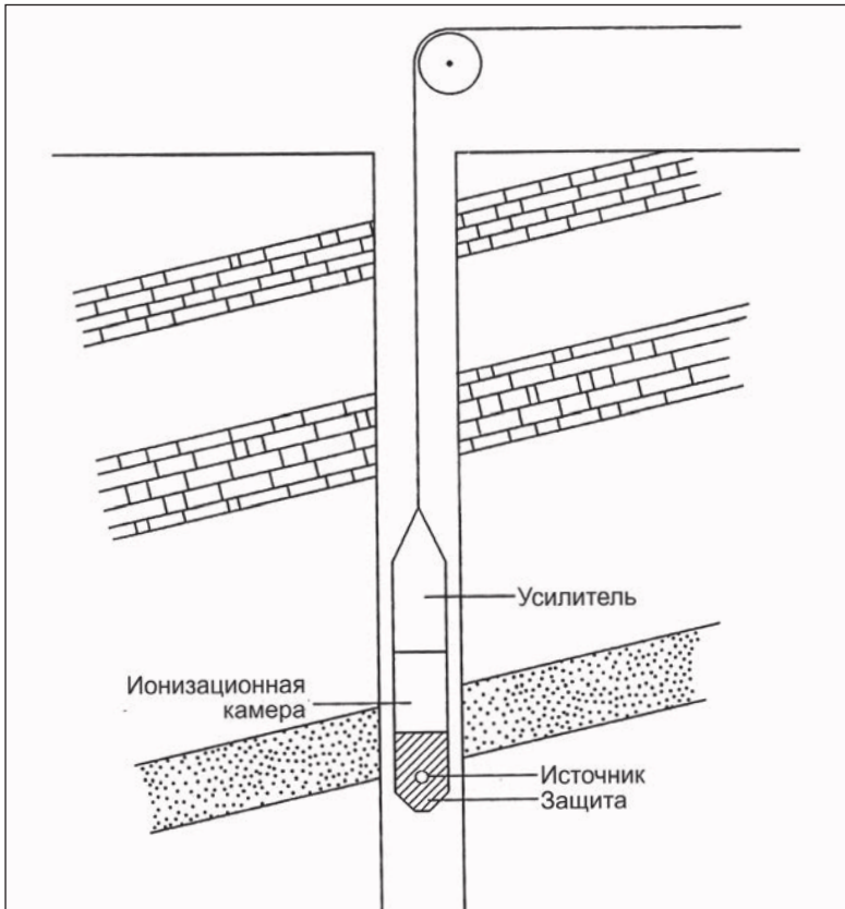
Схема расположения различных компонентов подземного оборудования относительно источника нейтронов
